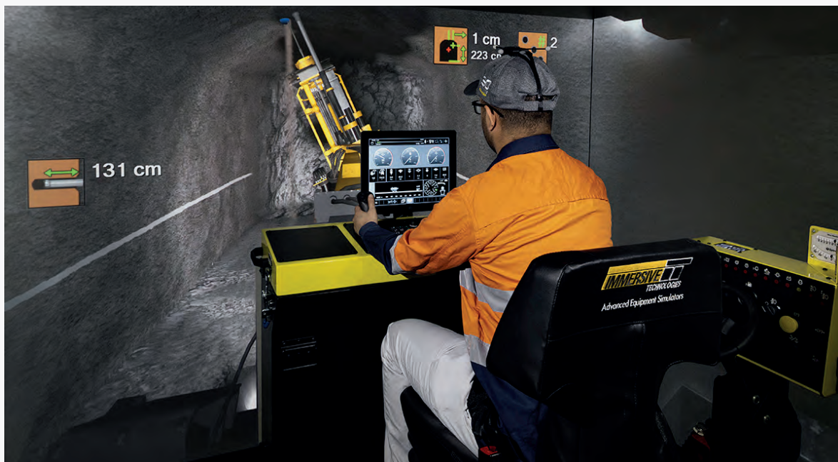
Simulateur de pointe IM360+ équipé d'un Conversion Kit® pour perceuse de production Epiroc
